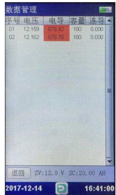
带连接电导测量的数据
